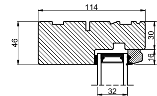
Lodret snit A
