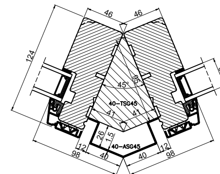
Udvendig hjørne 45° / External corner 45°
