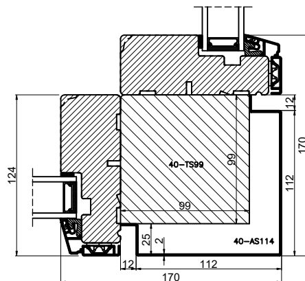
Udvendig hjørne 90° / External corner 90°
