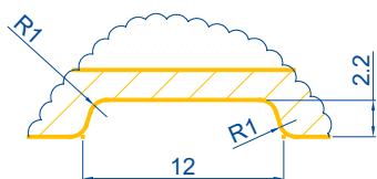
Dør-spor
