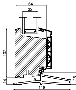
Med glasfibertrin
