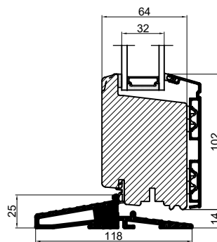
Med alutrin
