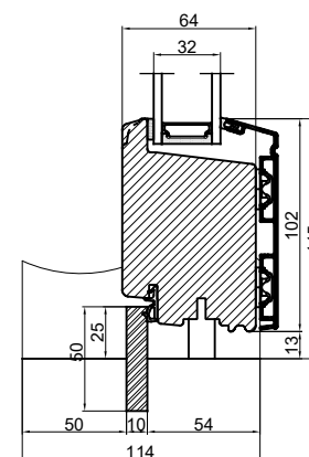
Med jernbundskinne
