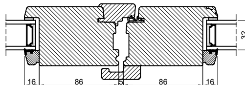
Vandret snit B
