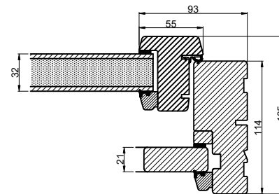
Vandret snit B
