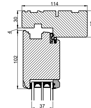
Lodret snit B
