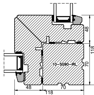
Udvendig hjørne 45° / External corner 45°
