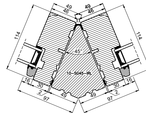
Udvendig hjørne 45° / External corner 45°
