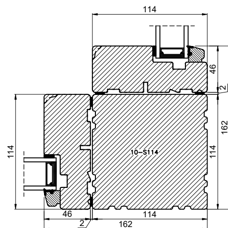
Udvendig hjørne 90° / External corner 90°
