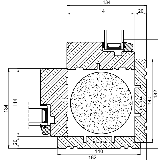
Udvendig hjørne / External corner
