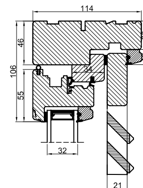
Lodret snit A
