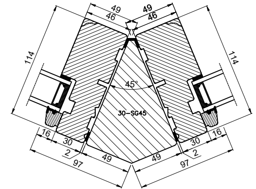
Udvendig hjørne 45° / External corner 45°
