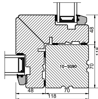
Udvendig hjørne 45° / External corner 45°
