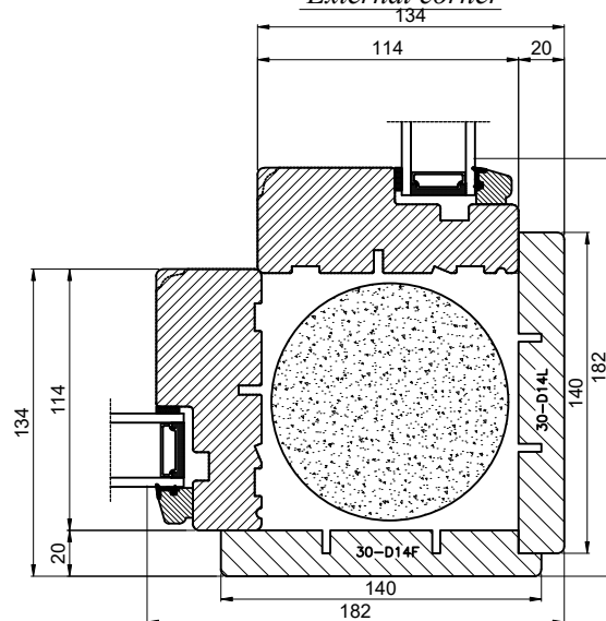
Udvendig hjørne / External corner
