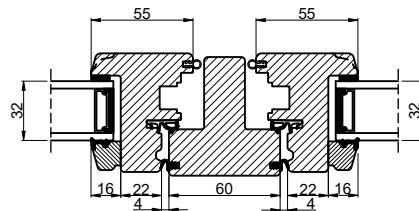
Vandret snit B
