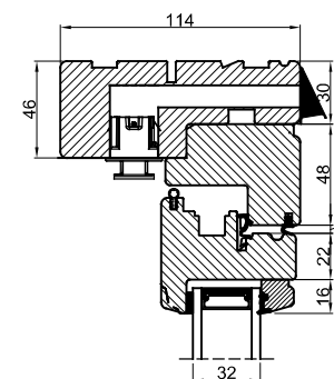
Indbygget kip-dreje indadgående
