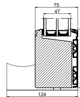
Uden trin
