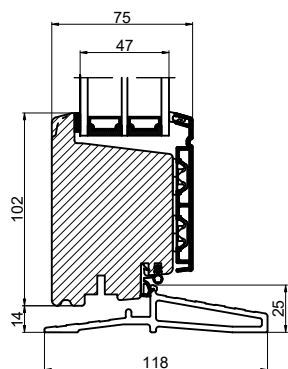
Med glasfibertrin
