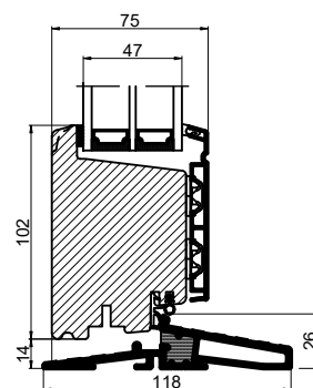
Med alutrin
