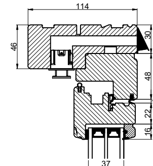
Indbygget dreje-kip indadgående
