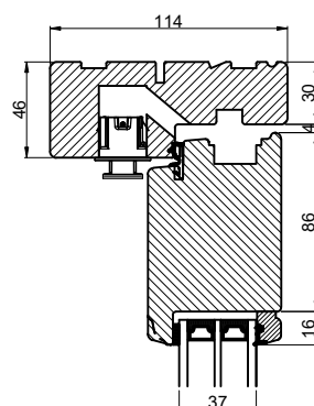
Udadgående dør
