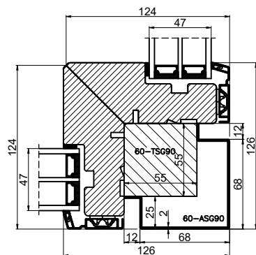
Udvendig hjørne 45° / External corner 45°
