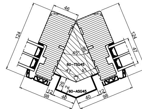
Udvendig hjørne 45° / External corner 45°
