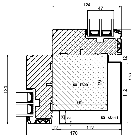
Udvendig hjørne 90° / External corner 90°
