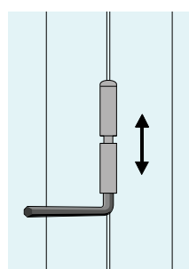
Figur 2: Justering af hængsel med en 5 mm unbrako
