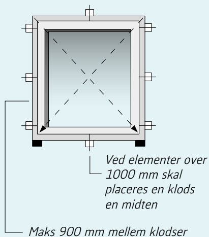
Figur 1: Krydsmål – tolerance +/- 2 mm
