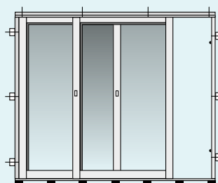
Figur 2: Eksempel med fastgørelsespunkter
