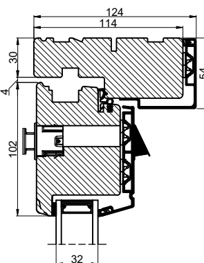
Indadgående dør
