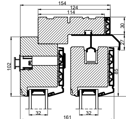
Hæveskydedør
