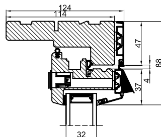
Kip-dreje indadgående
