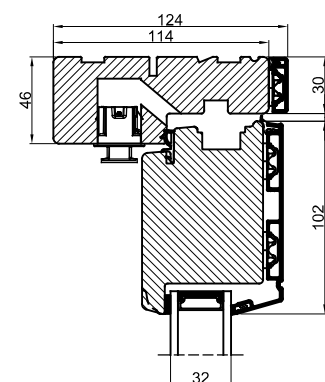
Udadgående dør
