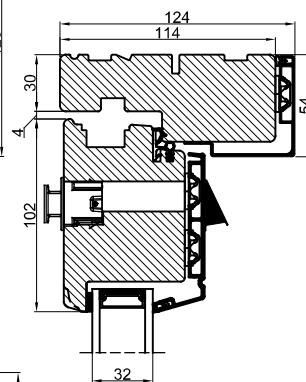
Indadgående dør
