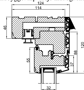
Kip-dreje indadgående
