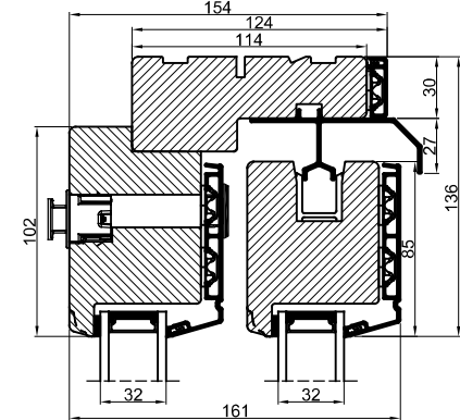
Hæveskydedør
