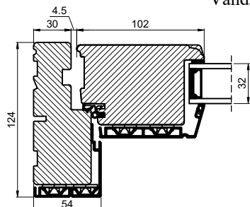
Vandret snit B
