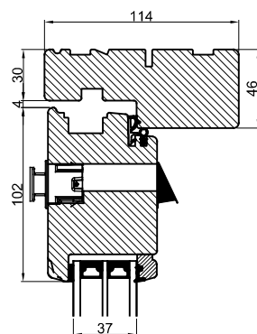
Indadgående dør
