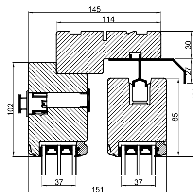
Hæveskydedør
