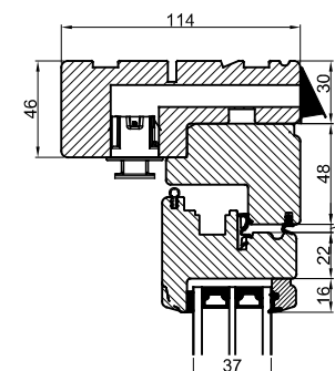
Kip-dreje indadgående
