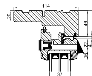
Kip-dreje indadgående
