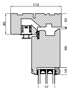
Udadgående dør
