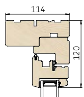
1 Lodret snit i overkarm/ramme
