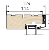
1 Lodret snit i overkarm
