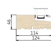
2 Lodret snit i bundkarm
