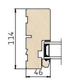
3 Vandret snit i sidekarm
