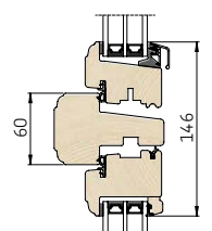
2 Lodret snit i vandret post/rammer
