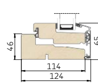
2 Lodret snit i bundkarm
