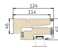
1 Lodret snit i overkarm/ramme
