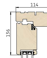
1 Lodret snit i overkarm/ramme
