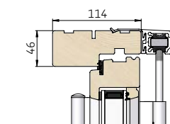
1 Lodret snit i overkarm/ramme
