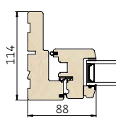
3 Vandret snit i sidekarm/ramme
