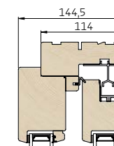
1 Lodret snit i overkarm/rammer
