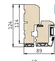
4 Vandret snit i sidekarm/ramme
