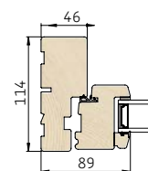
3 Vandret snit i sidekarm/ramme
