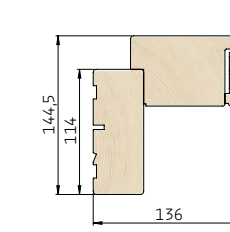
3 Vandret snit i sidekarm/ramme
