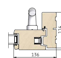
3 Vandret snit i sidekarm/ramme
