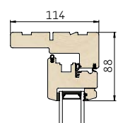
1 Lodret snit i overkarm/ramme
