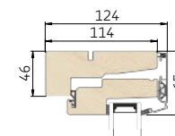
1 Lodret snit i overkarm/ramme
