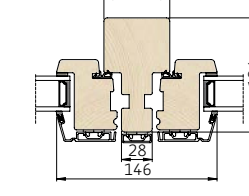
4 Vandret snit i lodpost/rammer
