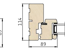
3 Vandret snit i sidekarm/ramme
