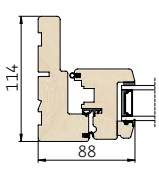
4 Vandret snit i sidekarm/ramme
