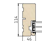
3 Vandret snit i sidekarm
