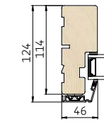
3 Vandret snit i sidekarm
