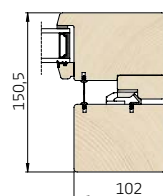
1 Lodret snit i overkarm/rammer
