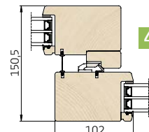
1 Lodret snit i overkarm/rammer
