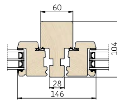
4 Vandret snit i lodpost/rammer
