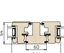
5 Vandret snit i lodpost/rammer
