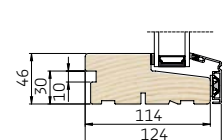
2 Lodret snit i bundkarm
