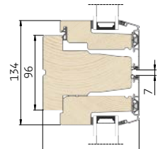
2 Lodret snit i vandret post/rammer
