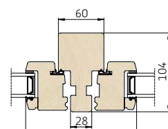
4 Vandret snit i lodpost/rammer
