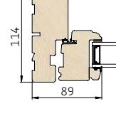
4 Vandret snit i sidekarm/ramme
