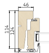
4 Vandret snit i sidekarm/ramme
