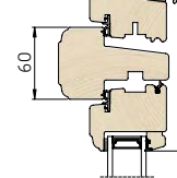
2 Lodret snit i vandret post/rammer
