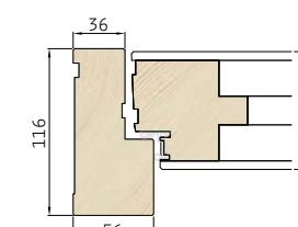
3 Vandret snit i sidekarm/ramme
