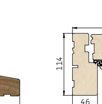
3 Vandret snit i sidekarm/ramme
