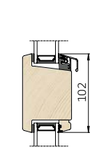
2 Lodret snit i tapstykke
