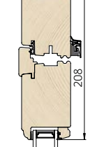
2 Lodret snit i midterrammer
