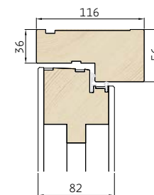
1 Lodret snit i overkarm/ramme
