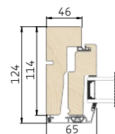
3 Vandret snit i sidekarme/rammer
