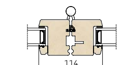
6 Vandret snit i sidekarm/ramme
