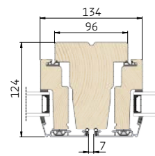
4 Vandret snit i lodpost/rammer
