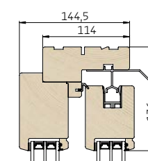
1 Lodret snit i overkarm/rammer
