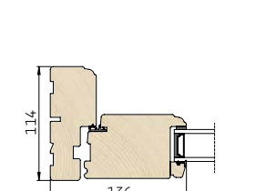
4 Vandret snit i sidekarm/ramme
