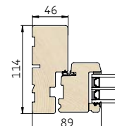
3 Vandret snit i sidekarm/ramme
