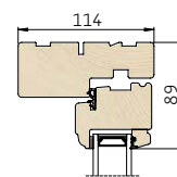
1 Lodret snit i overkarm/ramme
