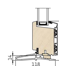
2 Lodret snit i bundkarm/spændestykke
