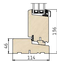
2 Lodret snit i bundkarm/spændestykke
