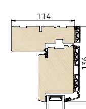
1 Lodret snit i overkarm/spændestykke
