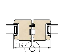
4 Vandret snit i rammer
