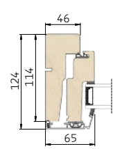
3 Vandret snit i sidekarm/ramme
