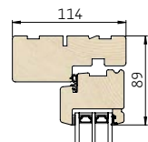
1 Lodret snit i overkarm/ramme
