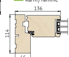
3 Vandret snit i sidekarm/ramme
