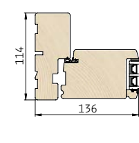
4 Vandret snit af sidekarm/ramme
