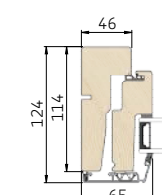
3 Vandret snit i sidekarm/ramme
