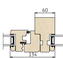
4 Vandret snit i lodpost/ramme
