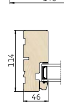
3 Vandret snit i sidekarm
