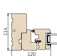
3 Vandret snit i sidekarm/ramme
