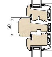
2 Lodret snit i vandret post/rammer
