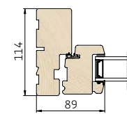
3 Vandret snit i sidekarm/ramme
