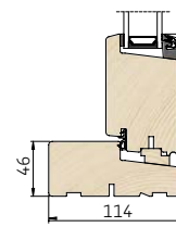
2 Lodret snit i bundkarm/spændestykke
