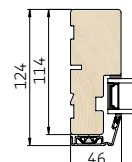
3 Vandret snit i sidekarm
