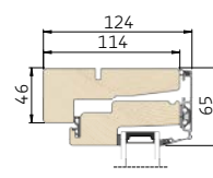
1 Lodret snit i overkarm/ramme
