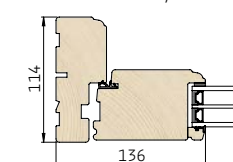
4 Vandret snit i sidekarm/ramme
