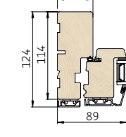
3 Vandret snit i sidekarm/ramme
